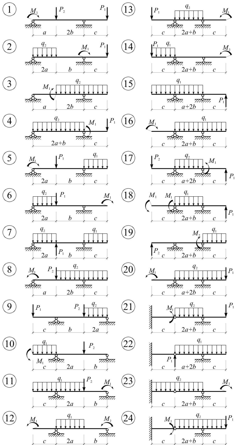
Рис.5.1 (Схемы балок для задачи №1)
